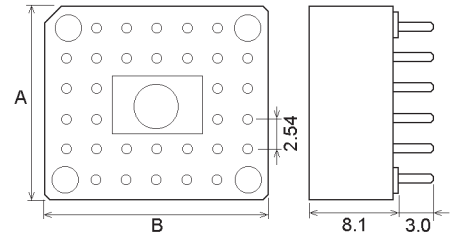
PLCC - 32 T-1
